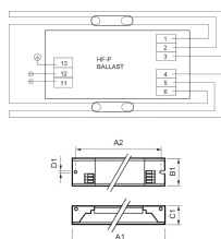
Technische Daten Philips HF-P 249 TL5 HO III 220-240V IDC für 2x49W
